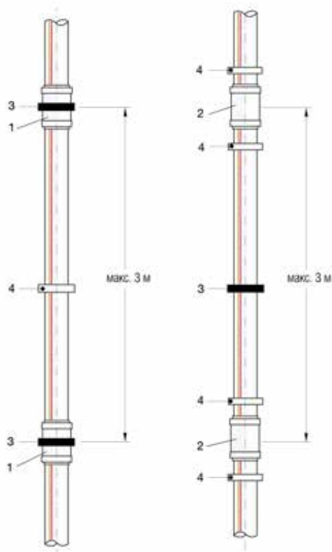
Рис. 76 Применение двухраструбных или подвижных муфт
